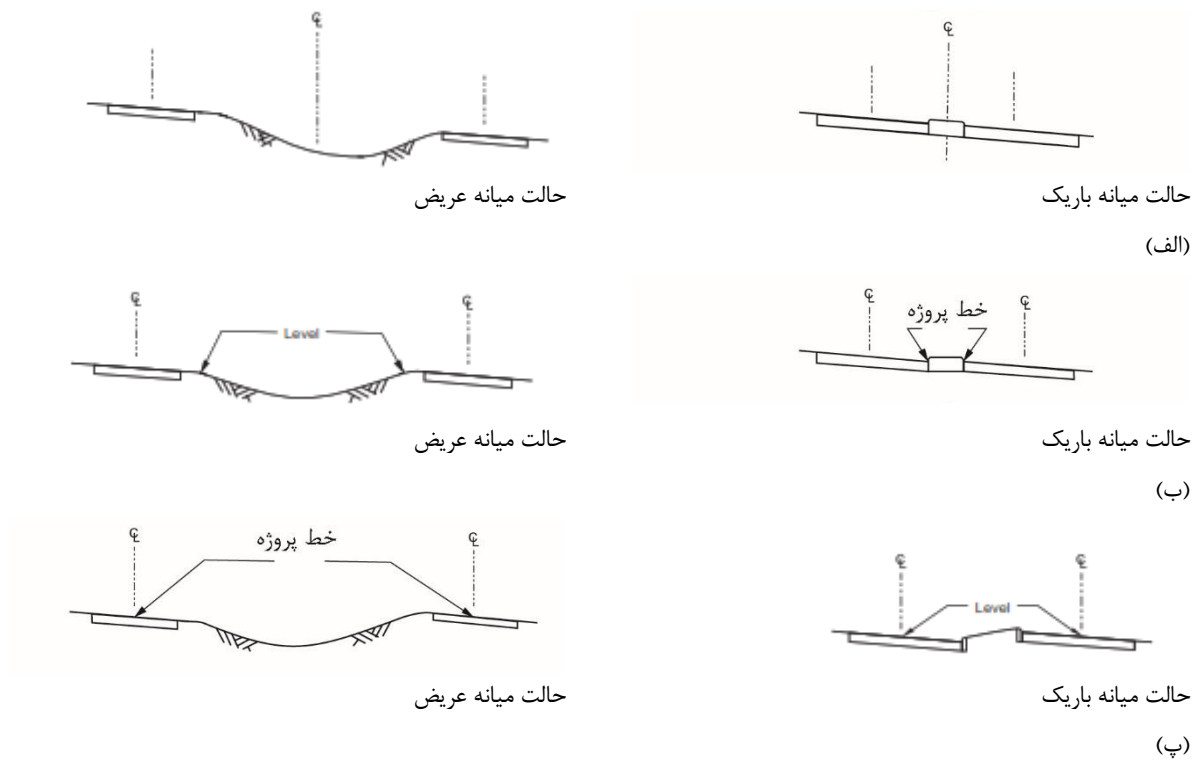
شکل ۵-۴- اعمال بریلندی در راه‌های مجزا
