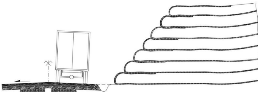
شکل ۶-۲۵ - خاک مسلح
