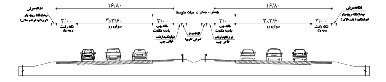
F11- آزادراه شش خطه با DDHV کمتر از ۲۵۰ با میانه متوسط
