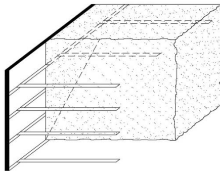
شکل ۶-۲۵ - خاک مسلح
