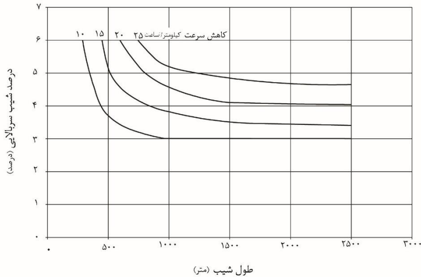
شکل ۵-۱۴- طول بحرانی شیب طولی برای وسیله تفریحی تپ (سرعت اولیه ۹۰ کیلومتر بر ساعت)
