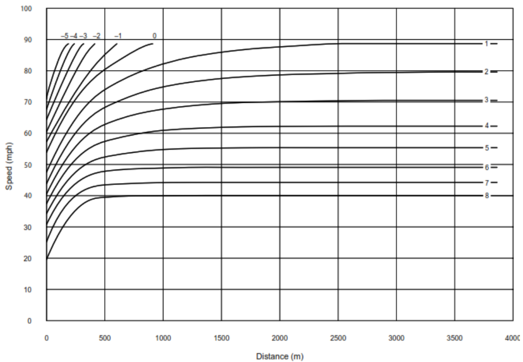
شکل ۵-۱۰ - منحنی سرعت - مسافت تریلی تیب سنگین ۱۴۰ پوند بر اسب بخار (۸۵ کیلوگرم بر کیلووات)
