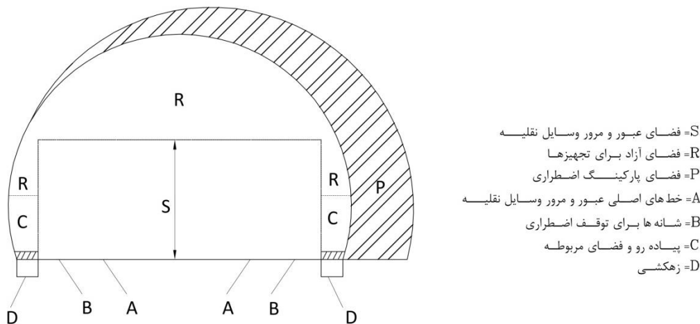
شکل ۶-۲۸- مقطع تونل به همراه پیاده‌روها، شانه‌ها، زهکشی و فضای ویژه توقف‌گاه (پارکینگ) اضطراری
