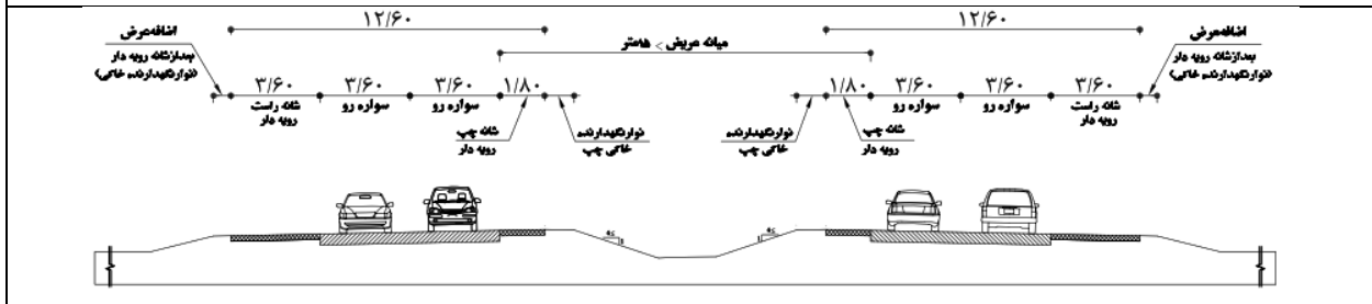
F10- آزادراه چهار خطه با DDHV برابر و بیشتر از ۲۵۰ با میانه عریض
