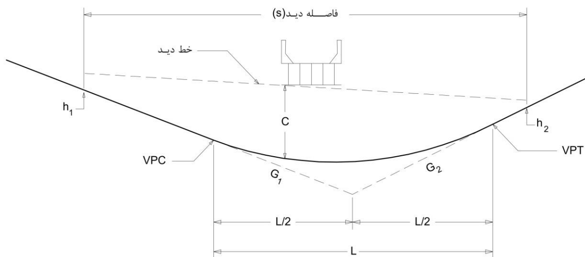
شکل ۵-۲۴- خط دید در خم کاسه‌ای
