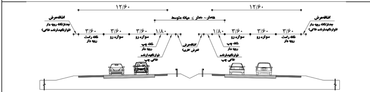
F9- آزادراه چهار خطه با DDHV برابر و بیشتر از ۲۵۰ با میانه متوسط
