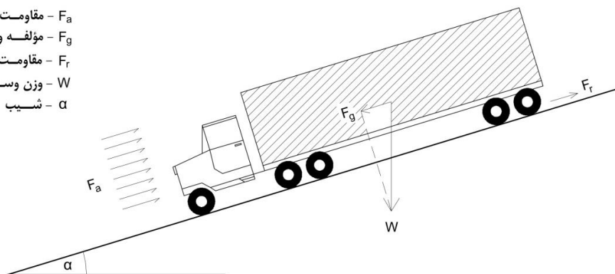
شکل ۵-۱۸- نیروهای وارده بر وسیله در حال حرکت در سرازیری
