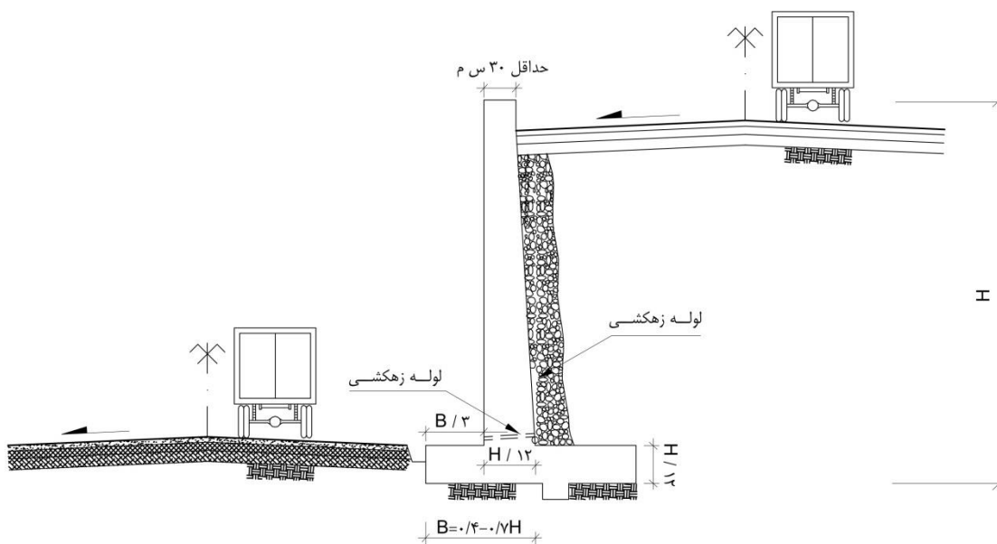
شکل ۶-۲۱- دیوار حائل وزنی
