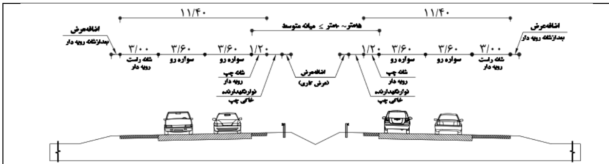
F7- آزادراه چهار خطه با DDHV کمتر از ۲۵۰ با میانه متوسط
