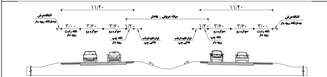
F8- آزادراه چهار خطه با DDHV کمتر از ۲۵۰ با میانه عریض
